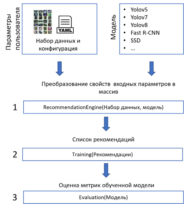
Принцип работы фреймворка для задач распознавания объектов
