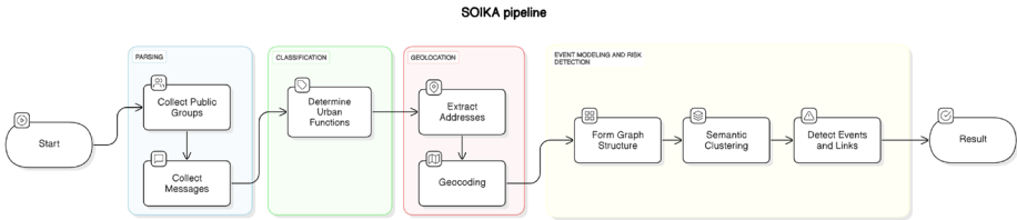
Схема работы модулей библиотеки: двухуровневая классификация, геолокация и обнаружение рисков
